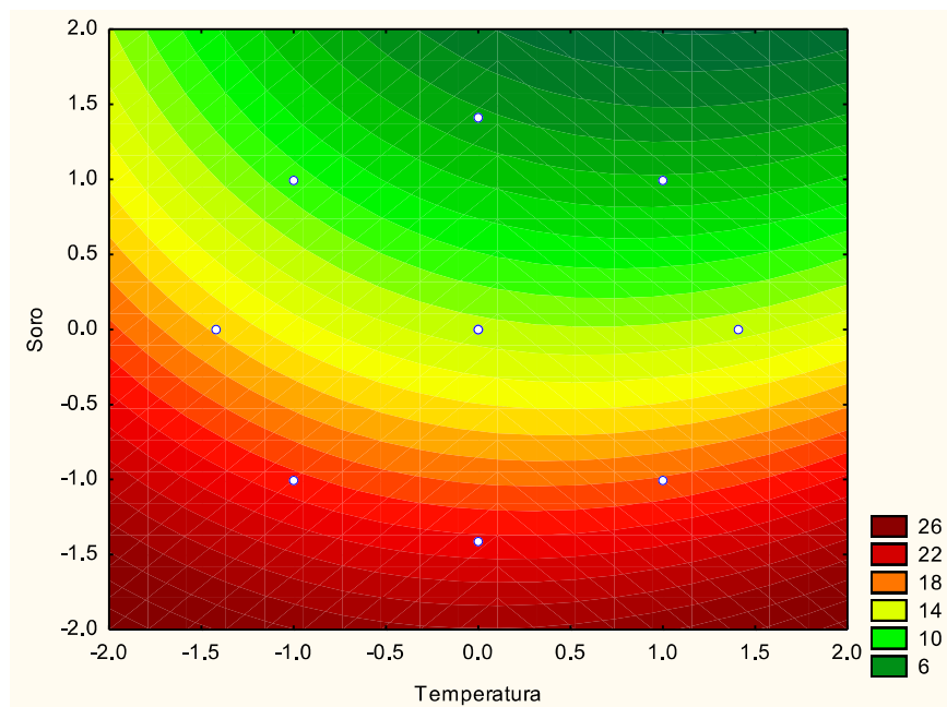
Figura 7. Curva de contorno da redução da tensão superficial em função da temperatura e diferentes concentrações de soro. F_{\text{calculado}} (9,54) > F_{\text{tabelado}} (5; 5; 0,05) = 5,05 , utilizando a ANOVA.
