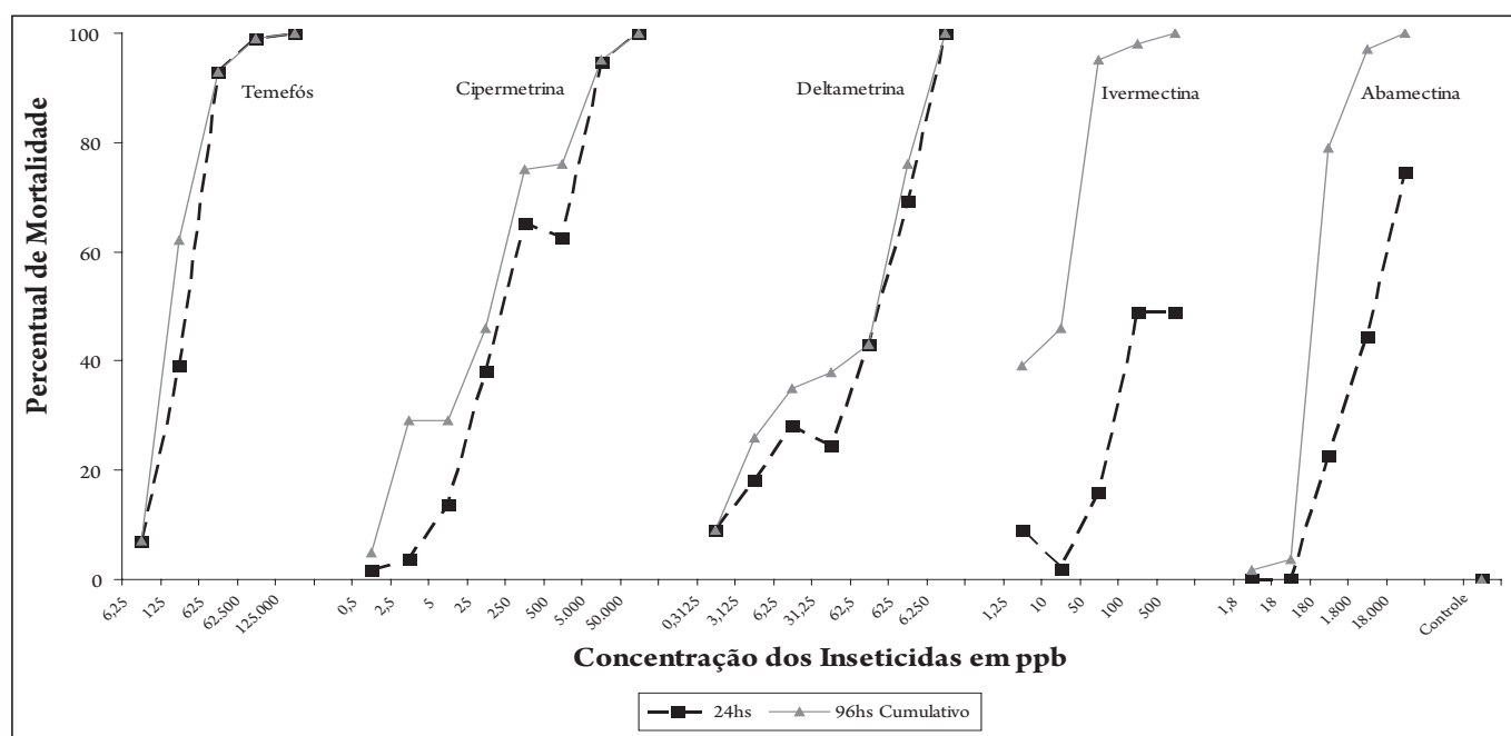
FIGURA 1 - Percentual de mortalidade por tempo de larvas de C. quinquefasciatus após 1h de exposição a diferentes concentrações de Inseticidas em ppb.
