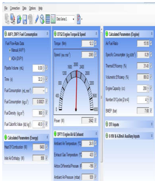
Fig.15: Modulo de Aquisição de Dados para MCI
