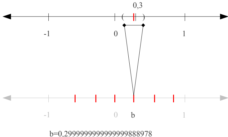
Figura 8: Representação do número 0,3 no computador com 64 bits. O “número” b representa um intervalo dos números reais, que inclui o valor 0,3. Os traços vermelhos representam pontos isolados.
