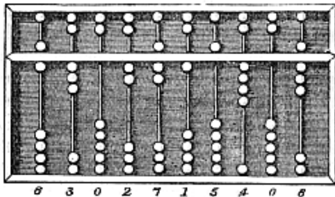
Figura 2: Representação do número 6302715408 em um ábaco . Fonte: Wikipédia.
