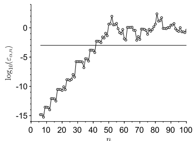
(b) Evolução do erro relativo (em logaritmo) \epsilon_{\alpha,n} da Eq. (16). Quando n \geq 44 o \epsilon_{\alpha,n} > \epsilon = \log_{10}(0,001) = -3 .
