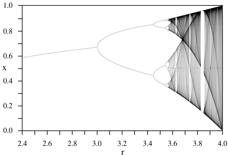
Figura 9: Diagrama de Bifurcação de (8). O eixo horizontal é o parâmetro r e o eixo vertical é o x . O valor inicial é x_0 = 0,25 . Fonte: Domínio Público.
