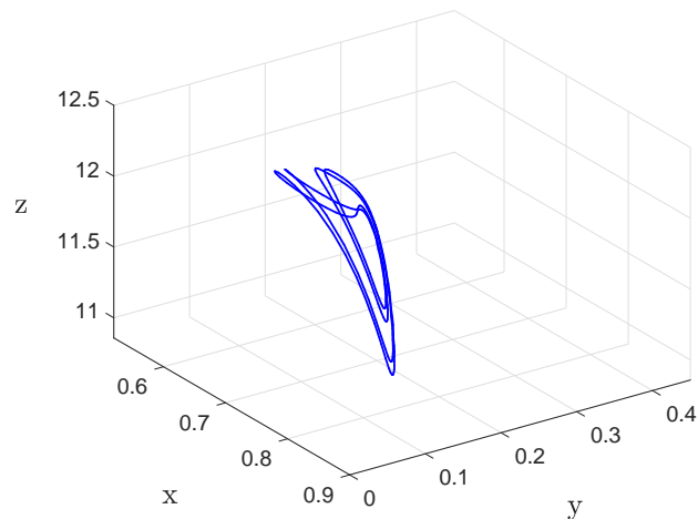
Figura 3.9: Ciclo limite de período 4 correspondendo ao parâmetro b_1 = 2,39 .
