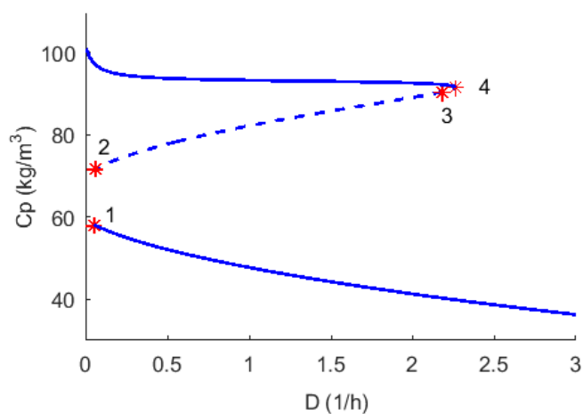
Figura 4.10: Diagrama de bifurcação da concentração de produto (etanol) em relação a taxa de diluição.
