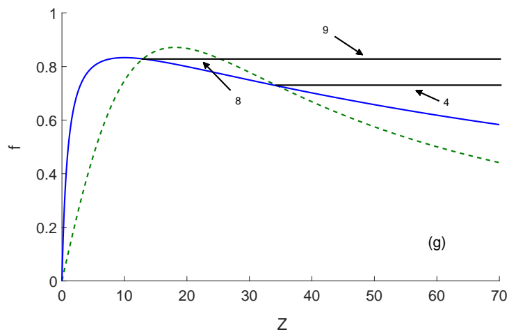
Figura 5.14: Diagrama operacional para os casos das curvas específicas da taxa de crescimento mostrado na Figura 5.7. O caráter dos estados estacionários em cada região do diagrama operacional são mostrados na Tabela 5.2.
