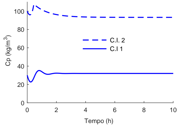
Figura 4.6: Concentração de produto (etanol) ao passar do tempo para C.I. 1 e 2
