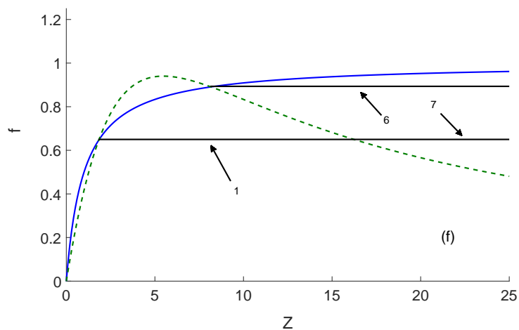
Figura 5.13: Diagrama operacional para os casos das curvas específicas da taxa de crescimento mostrado na Figura 5.6. O caráter dos estados estacionários em cada região do diagrama operacional são mostrados na Tabela 5.2.
