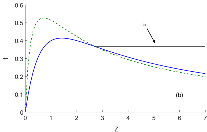
Figura 5.9: Diagrama operacional para os casos das curvas específicas da taxa de crescimento mostrado na Figura 5.2. O caráter dos estados estacionários em cada região do diagrama operacional são mostrados na Tabela 5.2.
