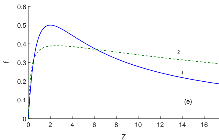
Figura 5.5: Curvas das taxas de crescimento específica das duas populações [Equações 5.8 e 5.9], sendo \alpha = 0.45 , \beta = 0.2 , \gamma_1 = 0.25 e \gamma_2 = 0.03
