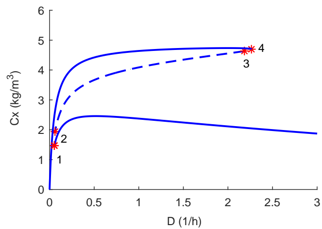
Figura 4.8: Diagrama de bifurcação da concentração de biomassa ( Z. mobilis ) em relação a taxa de diluição.
