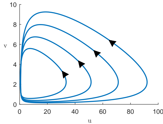
Figura 3.1: Soluções do modelo presa-predador de Lotka-Volterra, no plano de fase.
