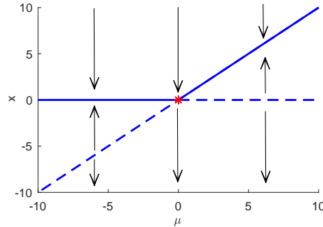
Figura 2.3: Bifurcação transcritical.
