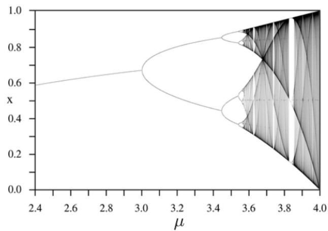
Figura 2.8: Bifurcação de duplicação de período "flip". Adaptado de [14]
