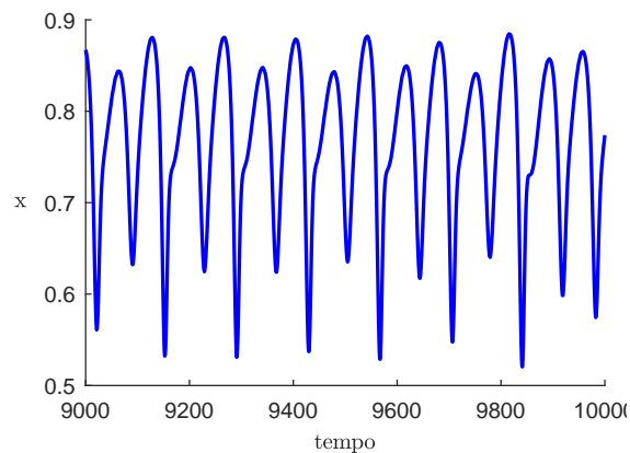
Figura 3.10: Espécie X ao passar do tempo com parâmetro b_1 = 2,39 .
