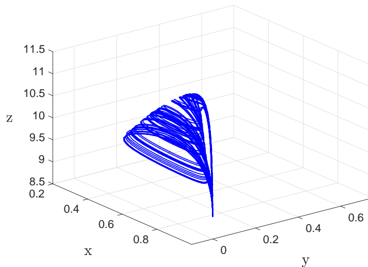
Figura 3.11: Um atrator caracterizado por comportamento caótico correspondendo ao parâmetro b_1 = 2,75 .
