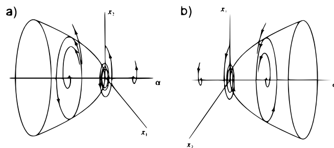
Figura 2.6: Bifurcação de Hopf: (a) subcrítica e (b) supercrítica. Retirado de [11]
