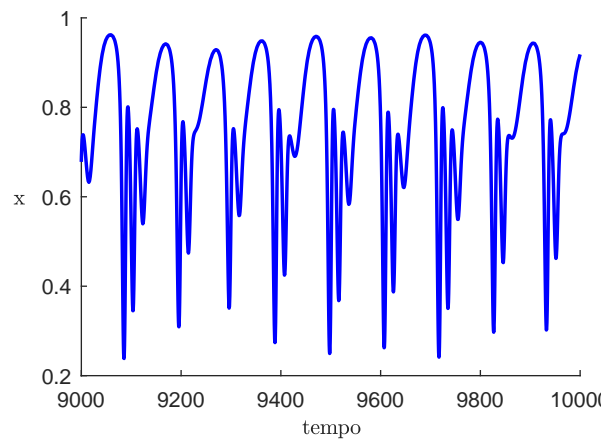
Figura 3.12: Espécie X ao passar do tempo, para o atrator que corresponde a b_1 = 2,75 .
