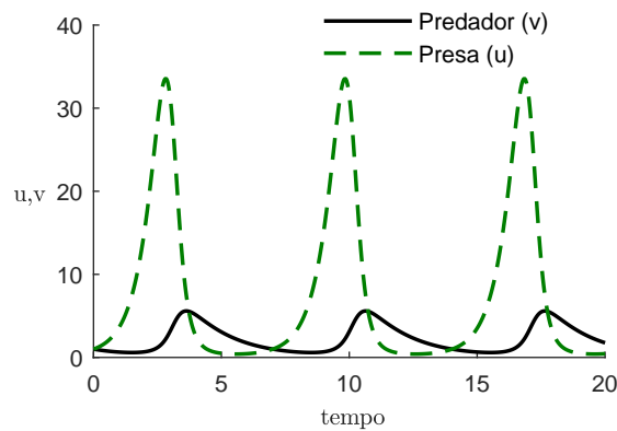
Figura 3.2: Densidade de presas e predadores ao passar do tempo
