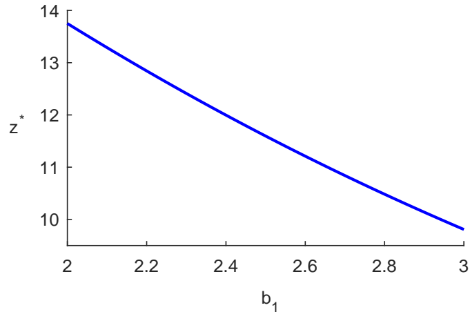
Figura 3.3: Valores de z^* variando o parâmetro b_1 no intervalo [2,3] .
